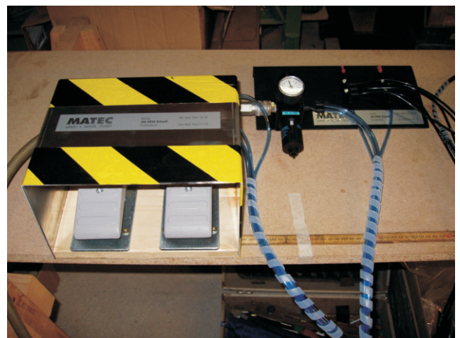
Fußschalter zur Bedienung der Rollen. Mit dem linken Pedal wird die erste und mit dem rechten die zweite Stufe bedient.
