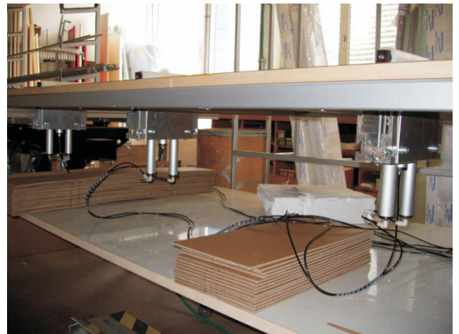
In der ersten Stufe lassen sich die Rollen um 60mm über die Arbeitsfläche anheben. Durch die Modulbauweise sind die Rollen praktisch überall einfach anzubringen.
